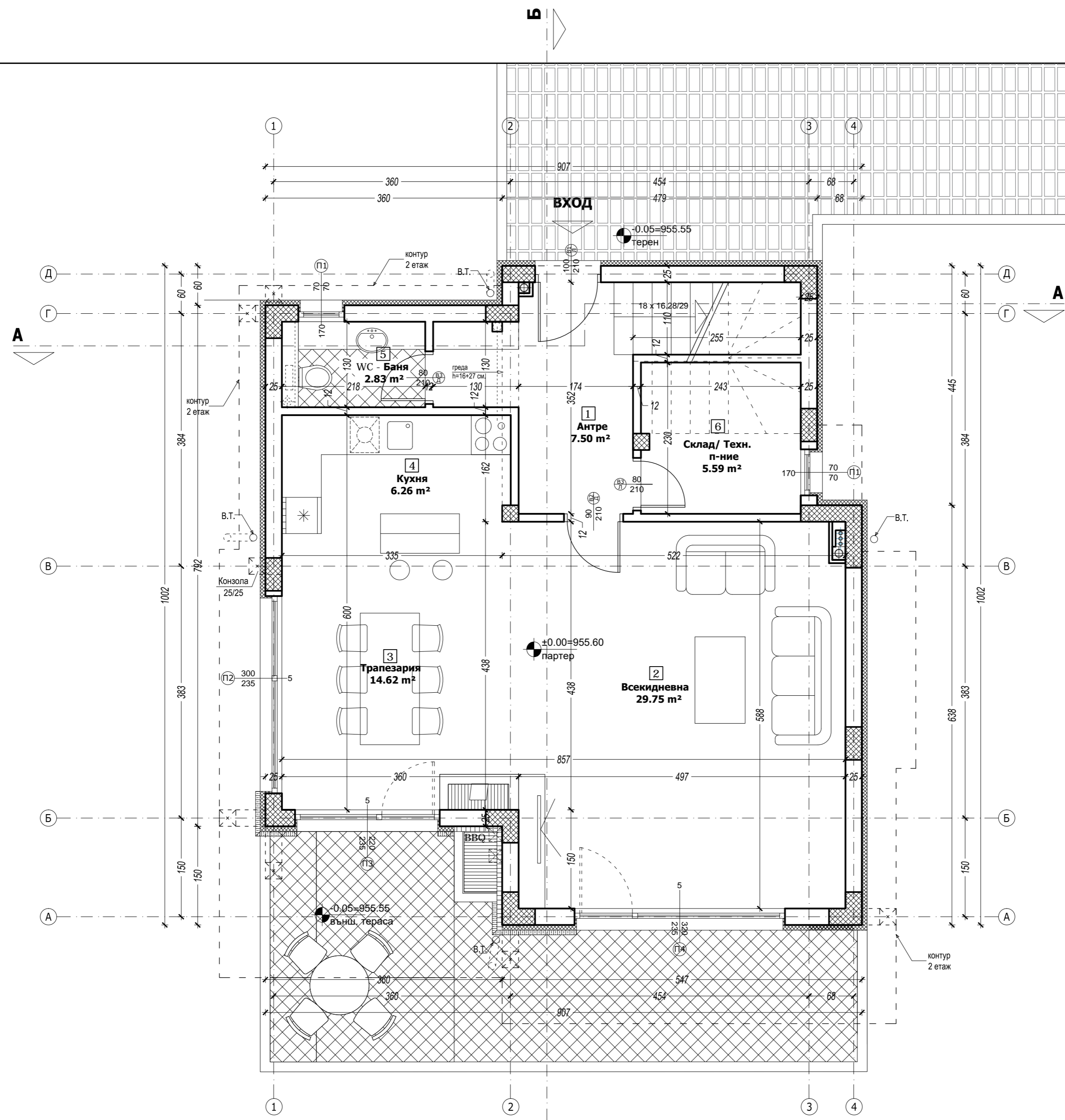
РАЗПРЕДЕЛЕНИЕ ПАРТЕР ПЛОЩ НА ЕТАЖА 83.93m 2
