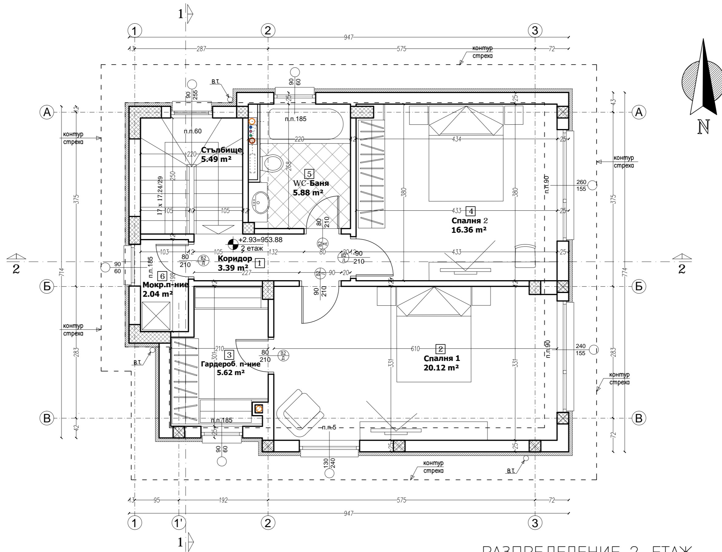
РАЗПРЕДЕЛЕНИЕ 2 ЕТАЖ ПЛОЩ НА ЕТАЖА 73.19 m 2
